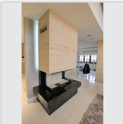
Spartherm Varia 3RL-100h-4s – wkład w zabudowie łączącej: dół wykonany z granitu polerowanego, góra ze szczotkowanego trawertynu. Całość z lekkim podświetleniem LED. Kratki wylotowe zastąpiono wnękami wykonanymi z kamienia w celu uniknięcia wprowadzenia kolejnego materiału i zachowania spójności. Również jest to wycinek kompletnego projektu wykończenia wnętrza.
